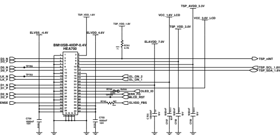
LCD Conector(MIPI)
