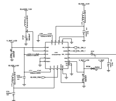
LCD DCDC
