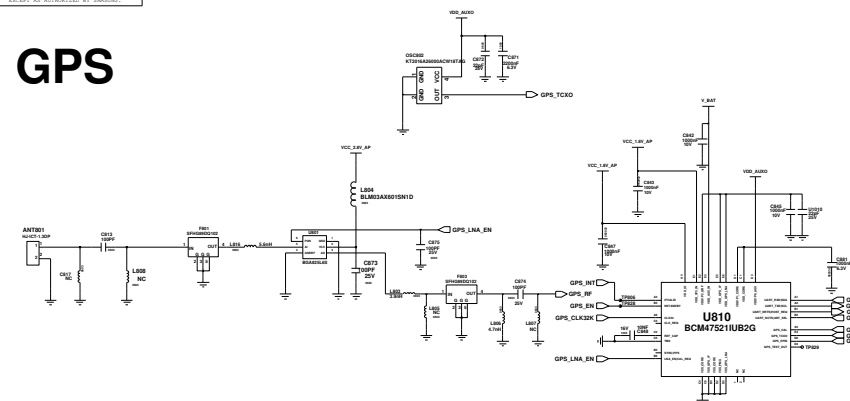
GPS(BCM47521)
